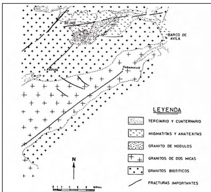
Tipos de rocas en la Sierra de Béjar J.M. Nieto y otros (1996), p.16
