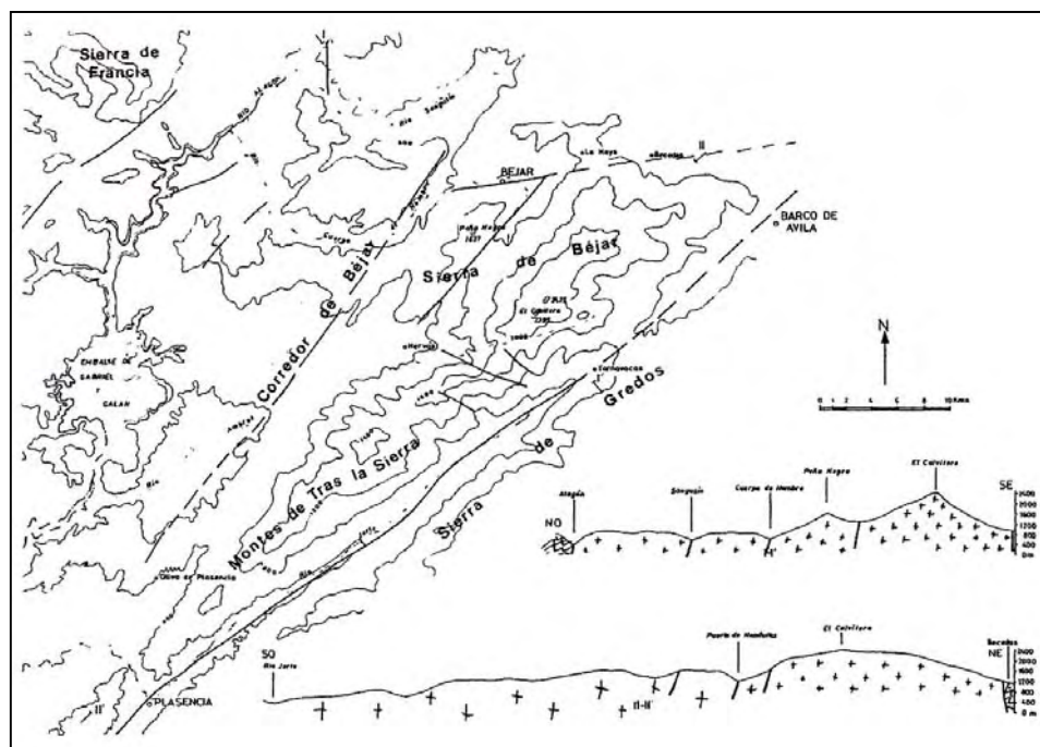
Esquema topográfico y morfológico de la Sierra de Béjar Según J.M. Nieto y otros (1996), p.14
